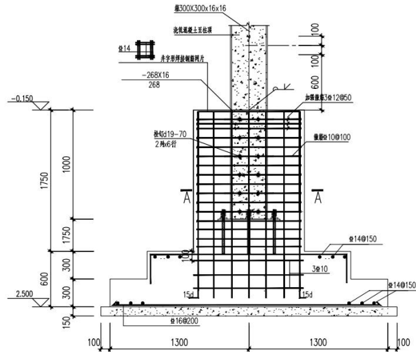
图 2.1-7 罩棚及加油岛基础平剖面图
