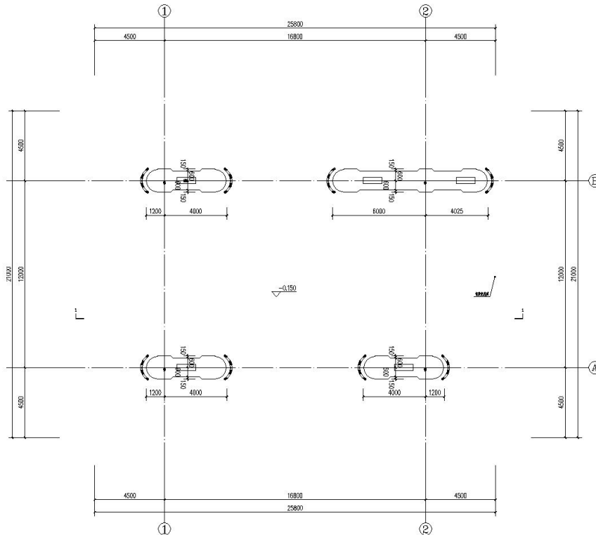
图 2.1-6 加油罩棚平面图 1: 100
