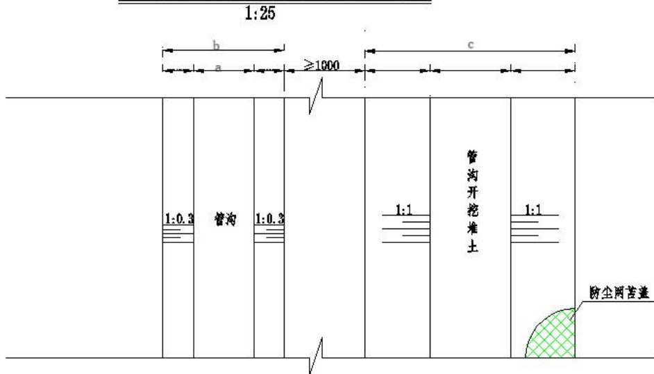
管道管沟开挖临时堆土临时防护剖面图
