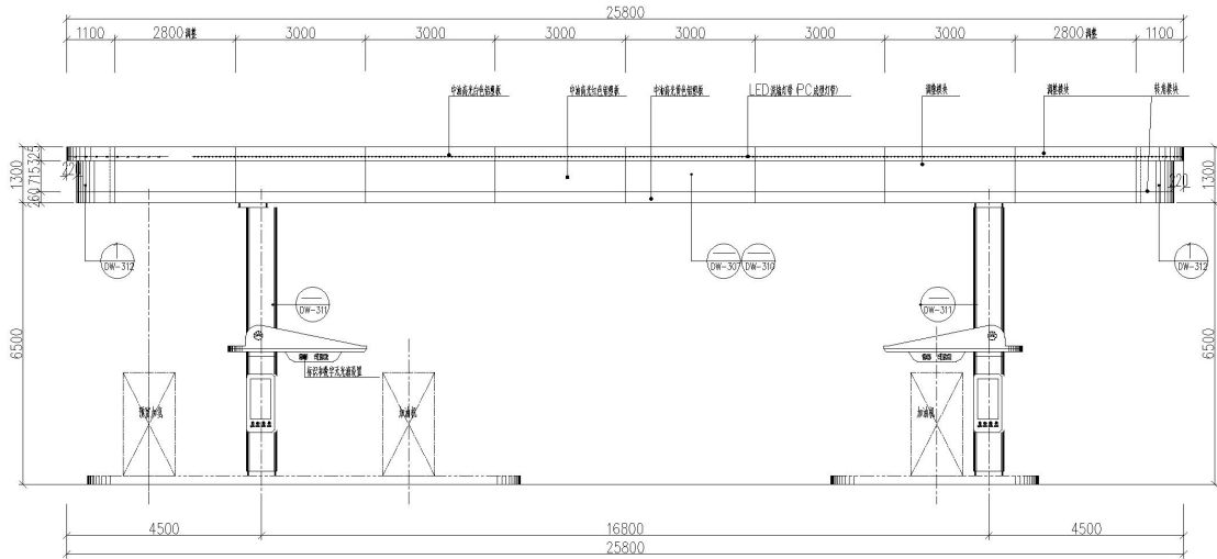
图 2.1-5 加油罩棚立面图 1: 100
