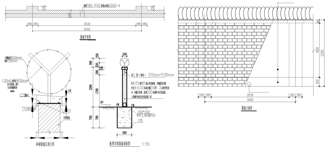
图 2.1-11 实体围墙平、立面图
