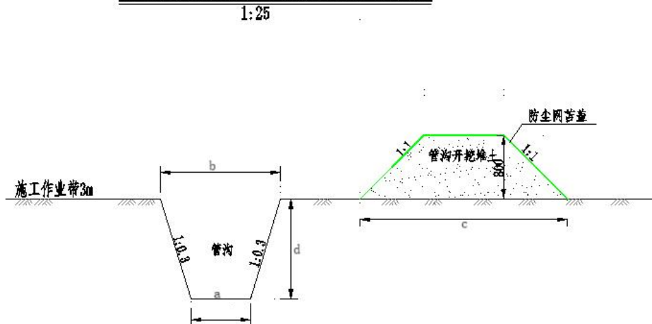
管道管沟开挖临时堆土临时防护剖面图
