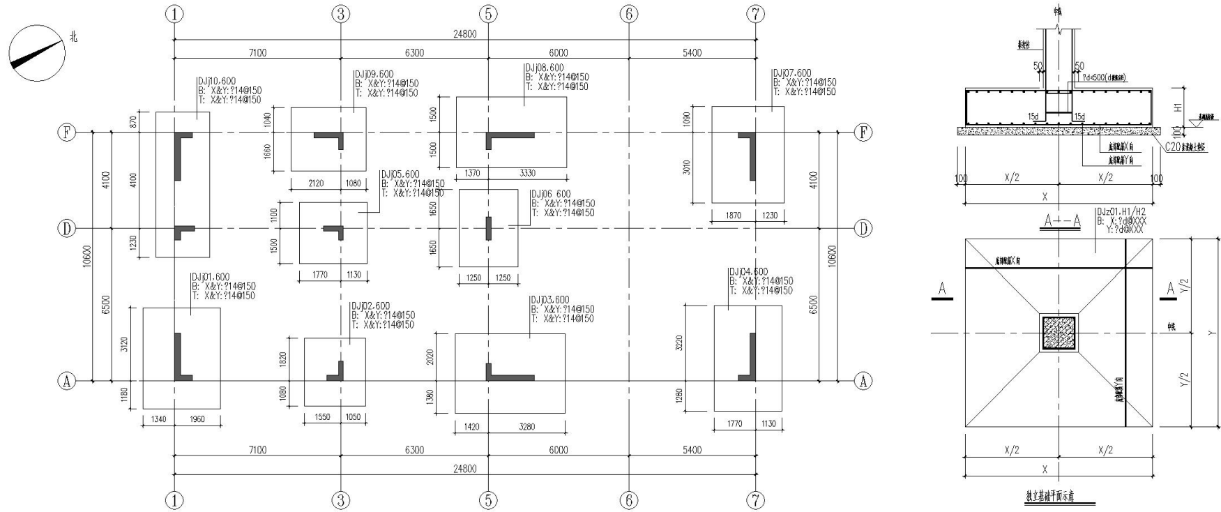
图 2.1-4 站房基础平剖面图 1: 100
