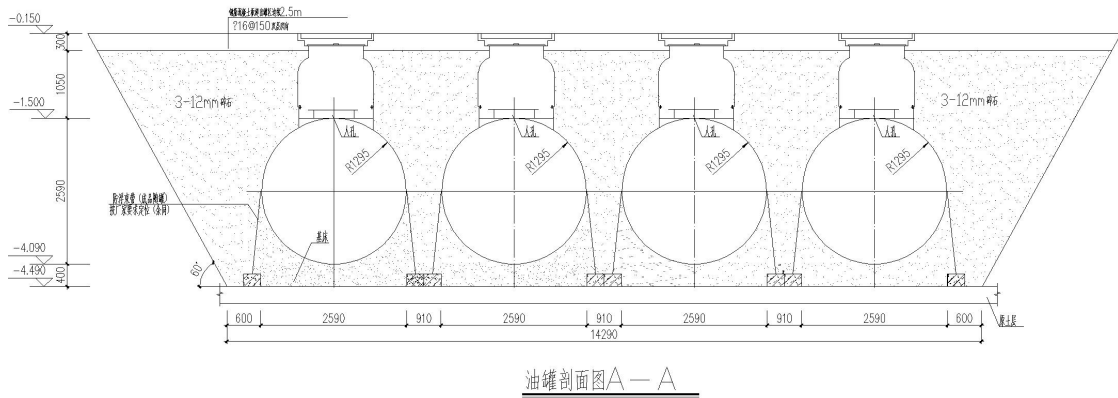
图 2.1-8 油罐剖面图 A-A
