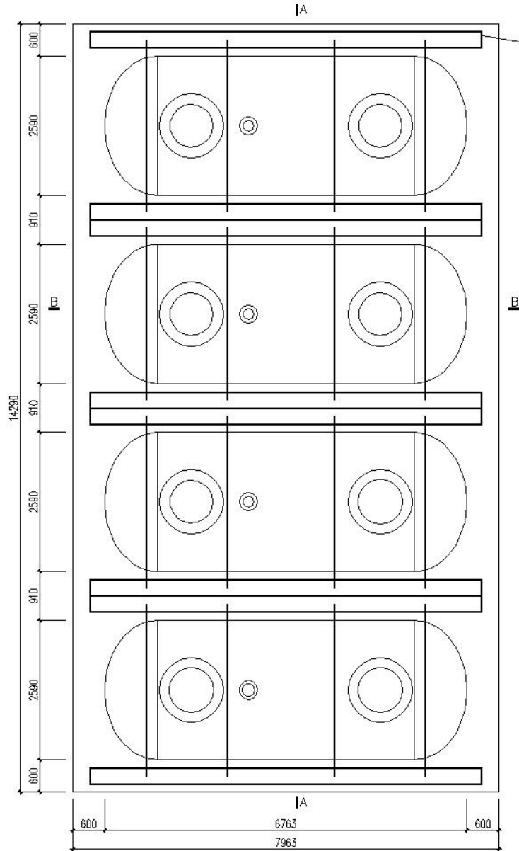
图 2.1-10 油罐平面图
