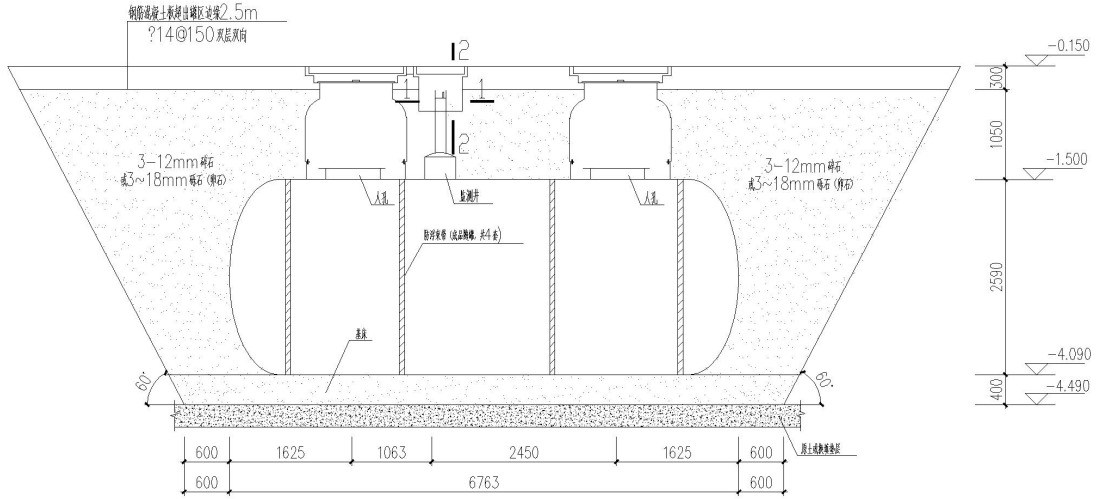
图 2.1-9 油罐剖面图 B-B
