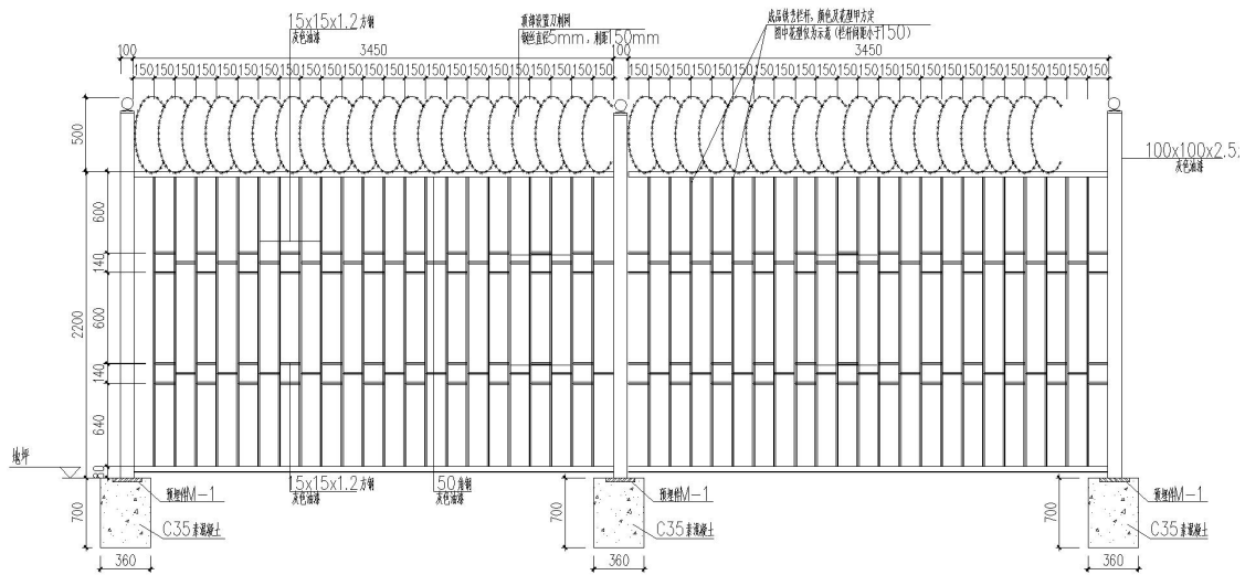
图 2.1-12 铁艺围墙平、立面图
