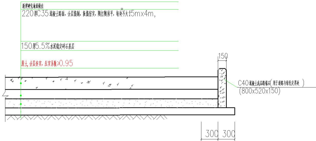
图 2.1-13 混凝土地坪铺砌详图
